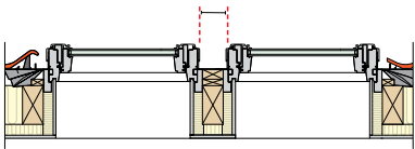
Bilden visar ett montage där befintlig takstol behålls.
